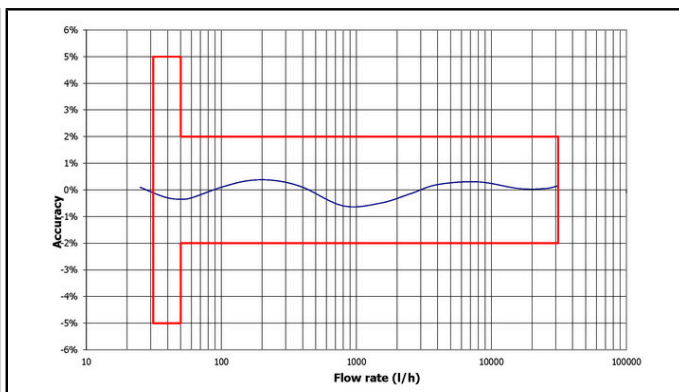
Typische Fehlerkurve - Q_3 25 m 3
